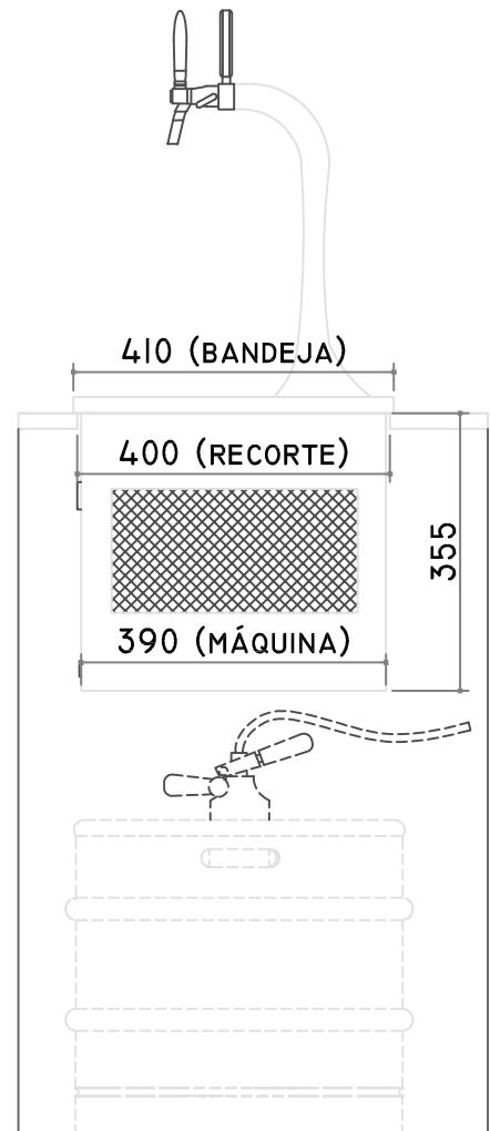
VISTA LATERAL
